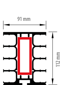
✓ 4-spurig Maximale Dachgröße 7000 x 5000 mm
